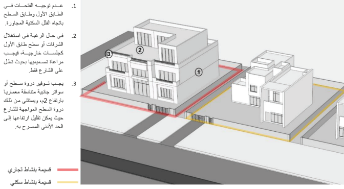
الشكل 2: الاشتراطات الخاصة بخصوصية الفلل السكنية المجاورة.
