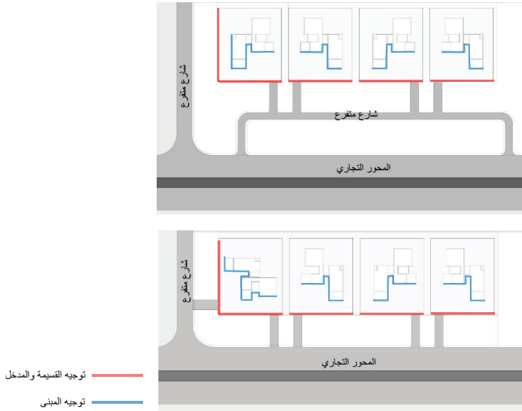
الشكل 1: التوجيه المسموح به للقسيمة والمبنى
